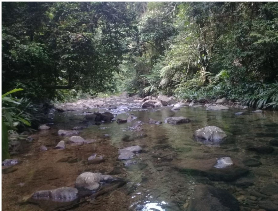
Mamóní 02. Zonas ribereñas (ríos, quebradas, etc.) dentro de los terrenos de la reserva (Foto: Nelson Guevara, 2021).
